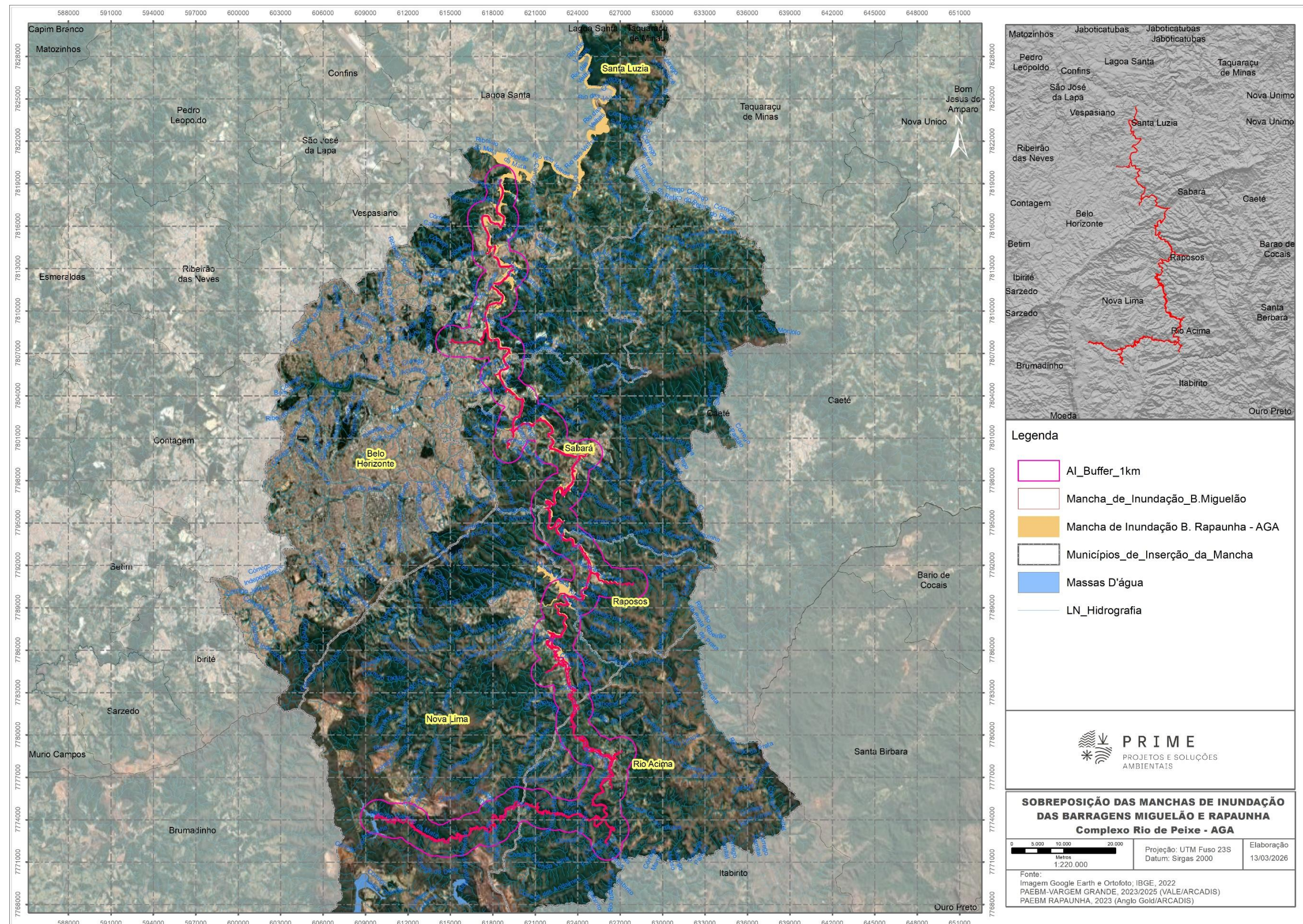
Figura 4 – Mapa de sobreposição das manchas de inundação das barragens Miguelão (AGA) e Rapaunha (AGA).
