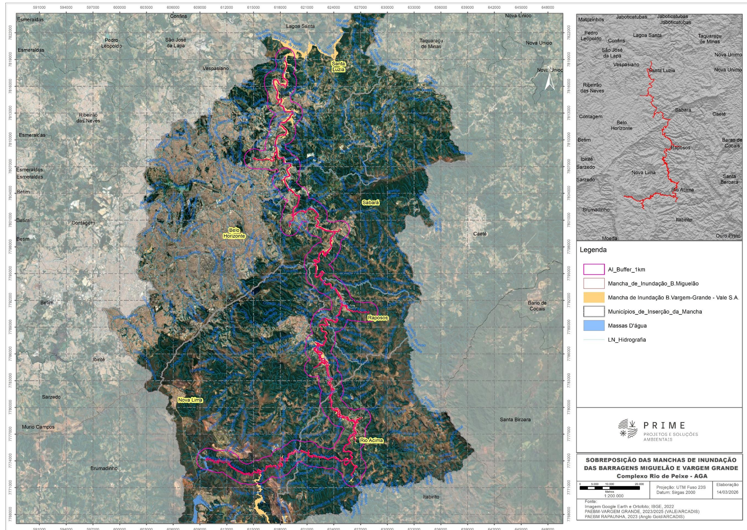
Figura 5 - Mapa de sobreposição das manchas de inundação das barragens Miguelão (AGA) e Vargem Grande (Vale S.A.)
