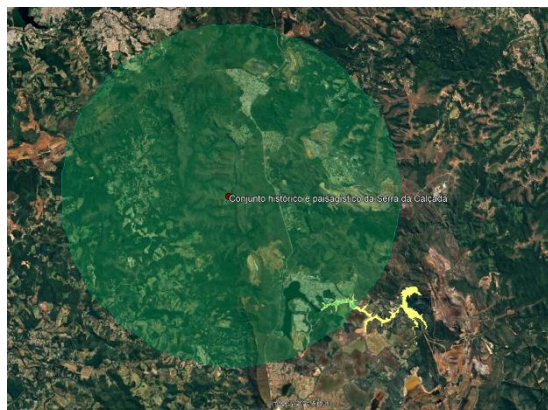
Figura 46. Interseção entre o raio de 10km (em verde) e a mancha de inundação (em amarelo). Elaboração: Prime, 2025.
